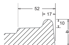
Edge profile
